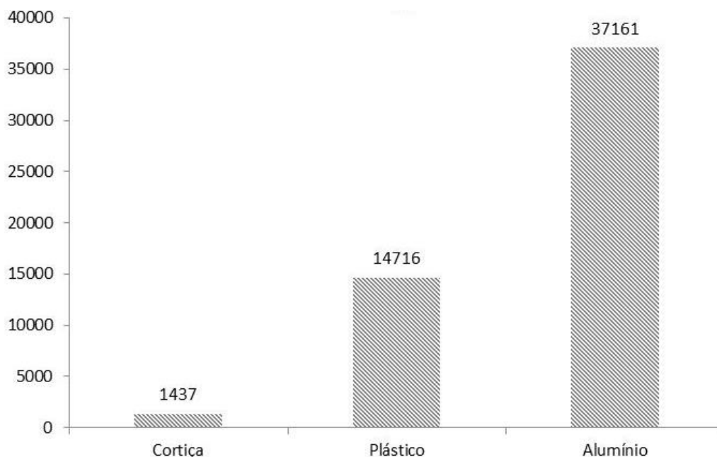
Gráfico 1 – Emissões de CO 2 (g)/1000 vedantes
